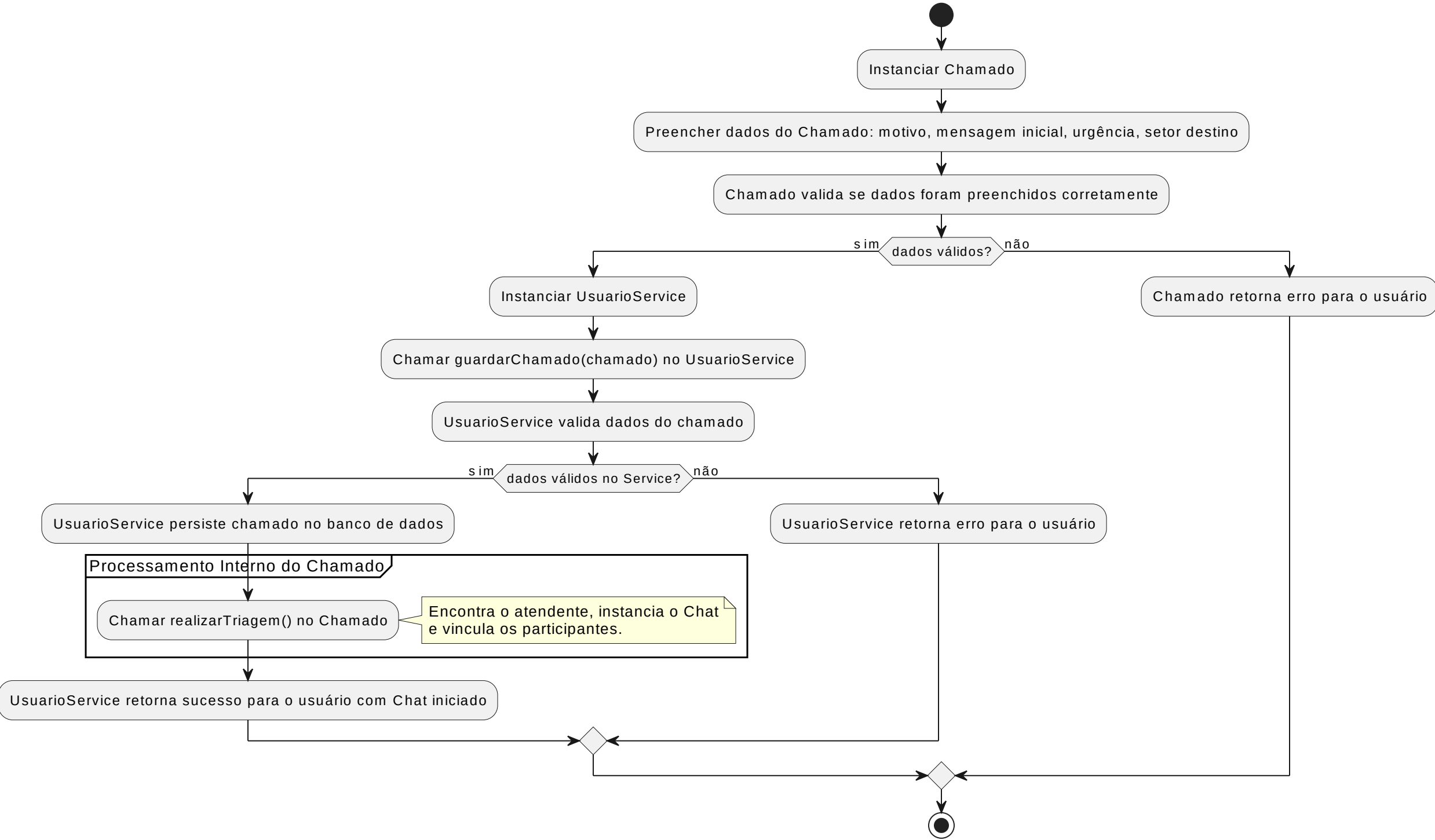
Diagrama de Atividade - Abrir Chamado (Fluxo Completo)
